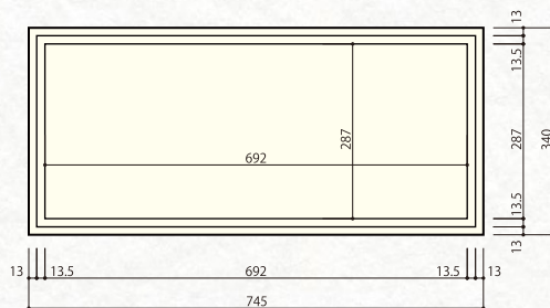
■ 上面図 s=1/10
