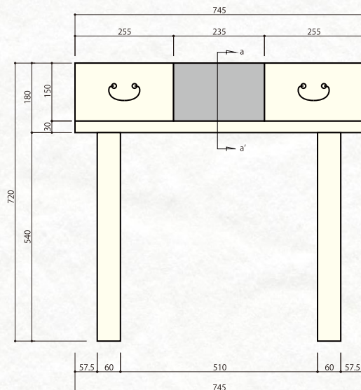
■ 正面図 s=1/10
