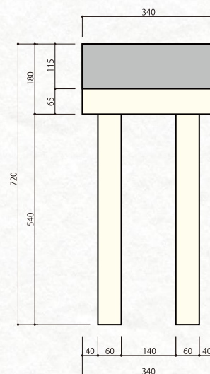
■ 側面図 s=1/10
